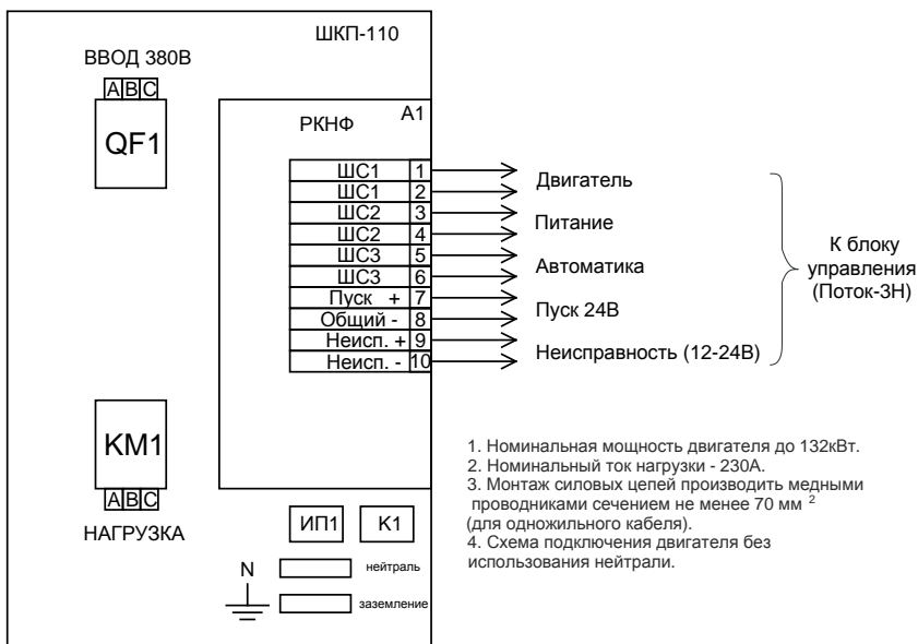
Рисунок 2. Схема электрического подключения шкафа ШКП-110 при эксплуатации
