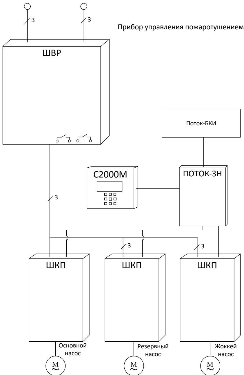
Рисунок 1. Схема питания ШКП в составе ПУ
